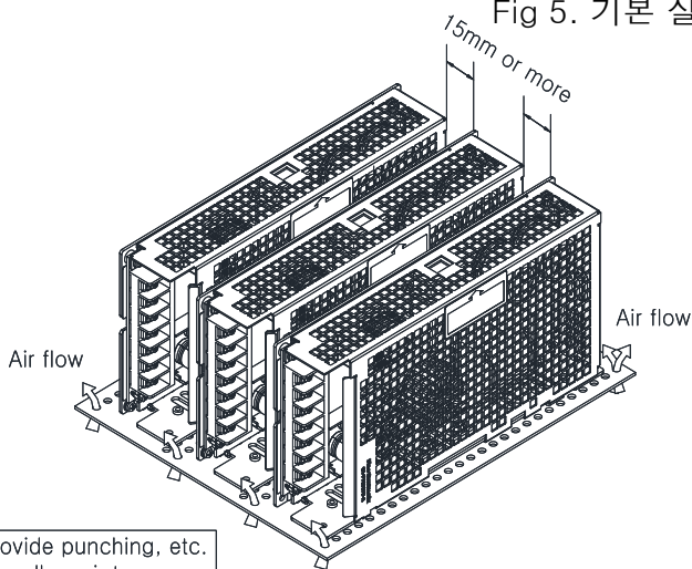
Fig 6. 응용 실장법
