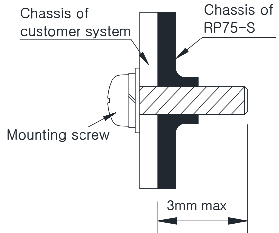
Fig 7. Screw 주의사항
