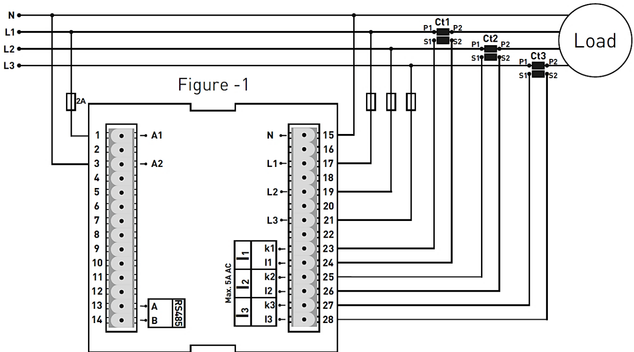
Figure-1: Kiểu kết nối 3P4W: Dòng điện ba pha và điện áp ba pha.
