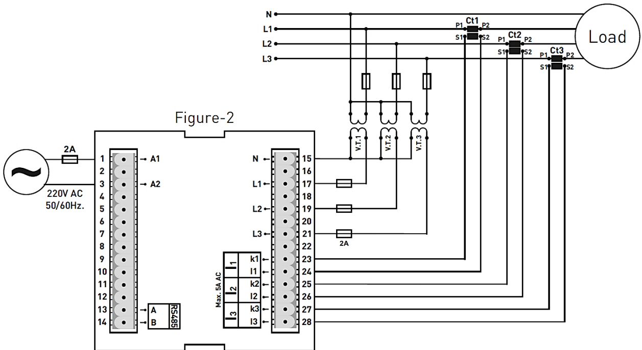
Figure-2: Dòng điện ba pha và điện áp ba pha. Phù hợp với trung áp, đi kèm biến áp.
