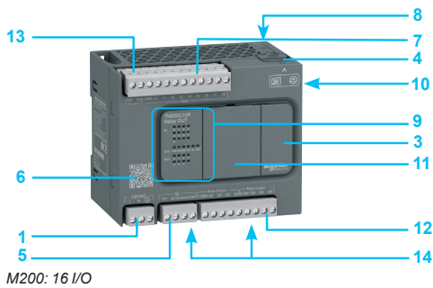
M200: 16 I/O
